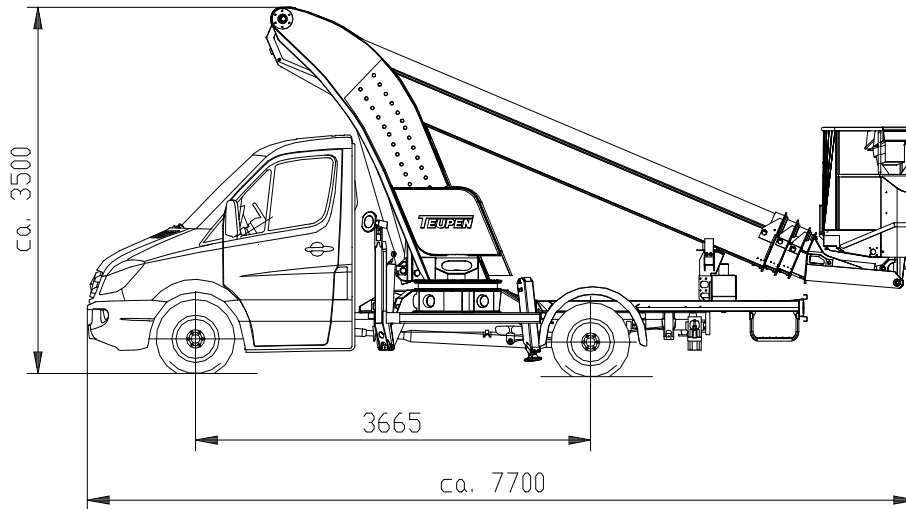
Beispiele Zugangstechnik Korbdrehen 180° - Korbanordnung aussermittigt
